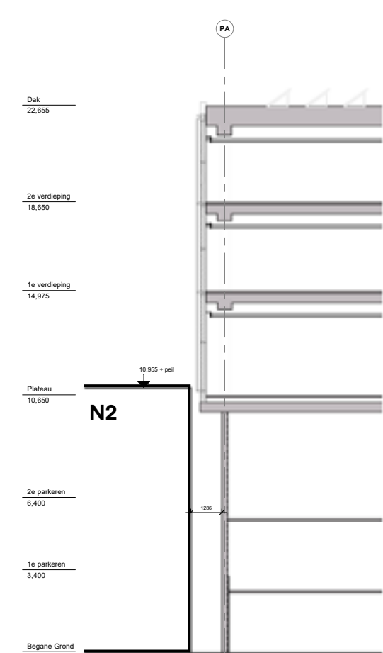
Zuid 2
