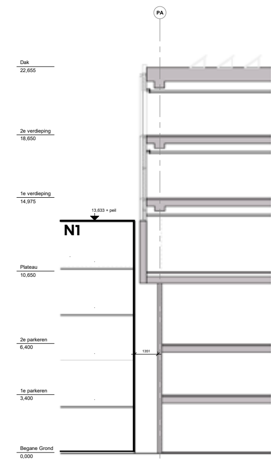
Zuid 1
